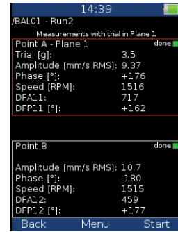
Auswuchten
